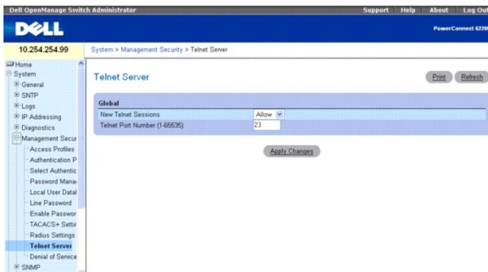
Ilustración 6-56. Servidor Telnet
